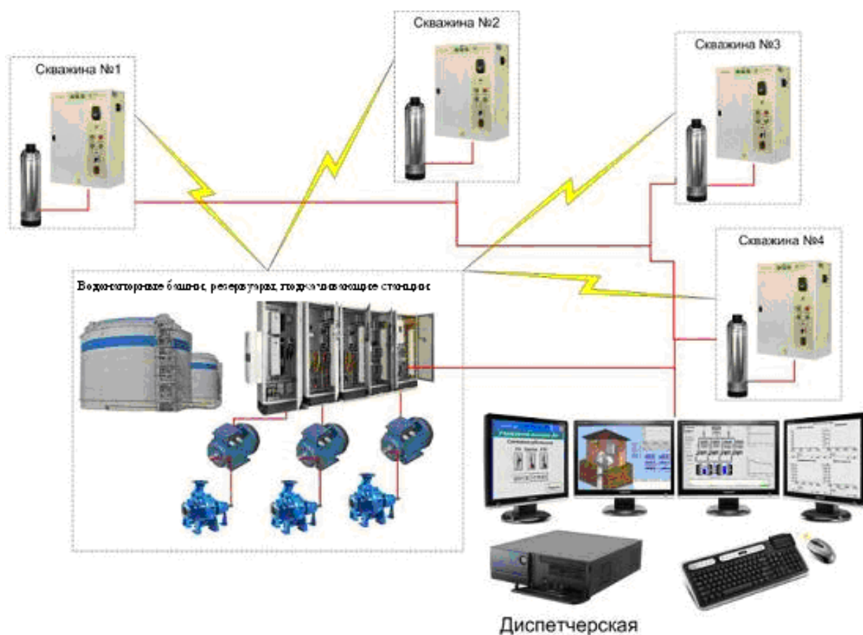
Рисунок 11 – Схема автоматизации, диспетчеризации и управления
