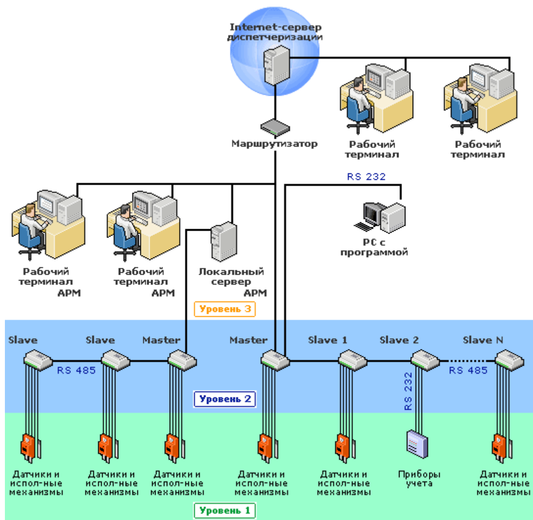
Рисунок 12 – Схема уровней системы АСУ ТП
