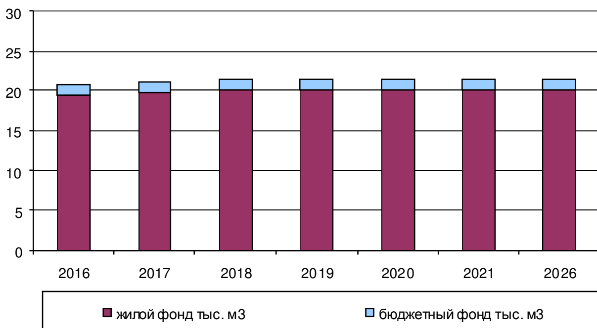
Рисунок 5 – Диаграмма перспективного баланса подачи и реализации воды по структурным составляющим
